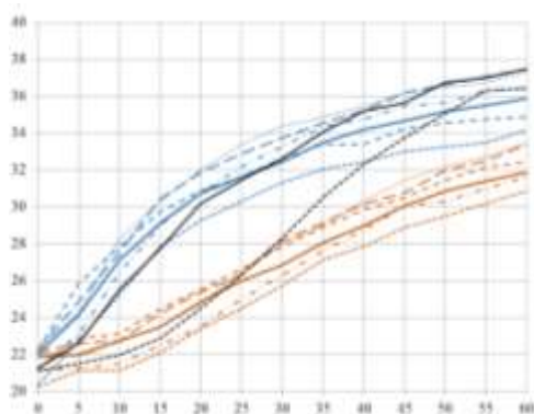
Сурет 2 - Әртүрлі сынақ сатыларындағы мотор-барабан бетінің температурасы
