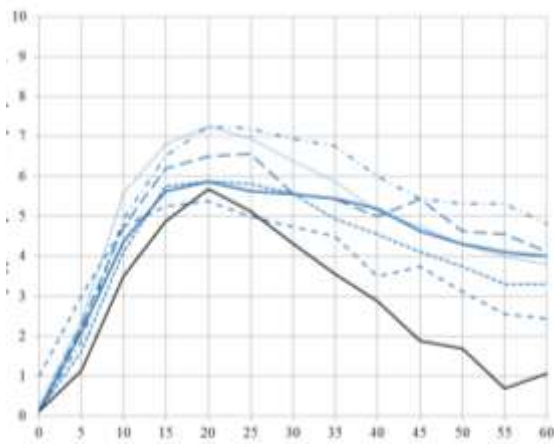
Сурет 4 - Мотор-барабан бетінің температурасы айырмашылықтарының шамасы сынақтардың әртүрлі сатыларында
