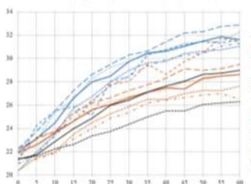
Сурет 3 - Әр түрлі сынақ сатыларындағы таспалар бұтақтарының беткі температурасы
